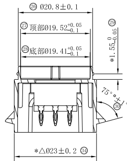
截面 A-A
