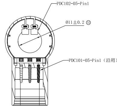
截面 C-C
