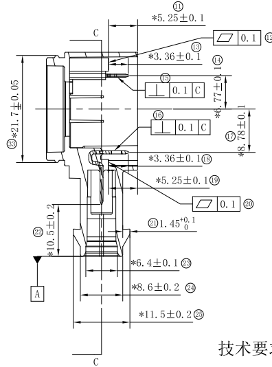
截面 B-B
