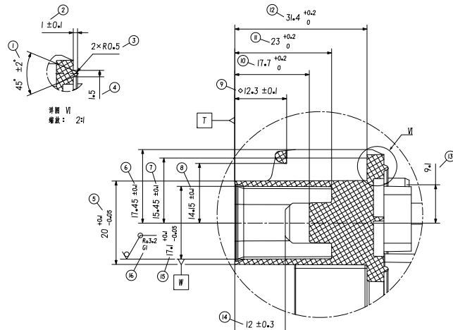
詳圖 I 縮放: 2x
