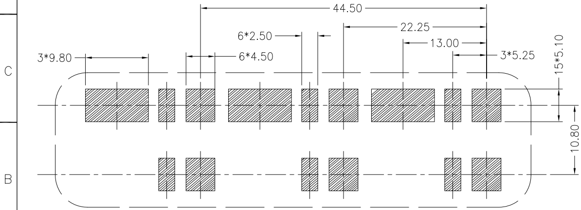
PCB 貼板參考尺寸
