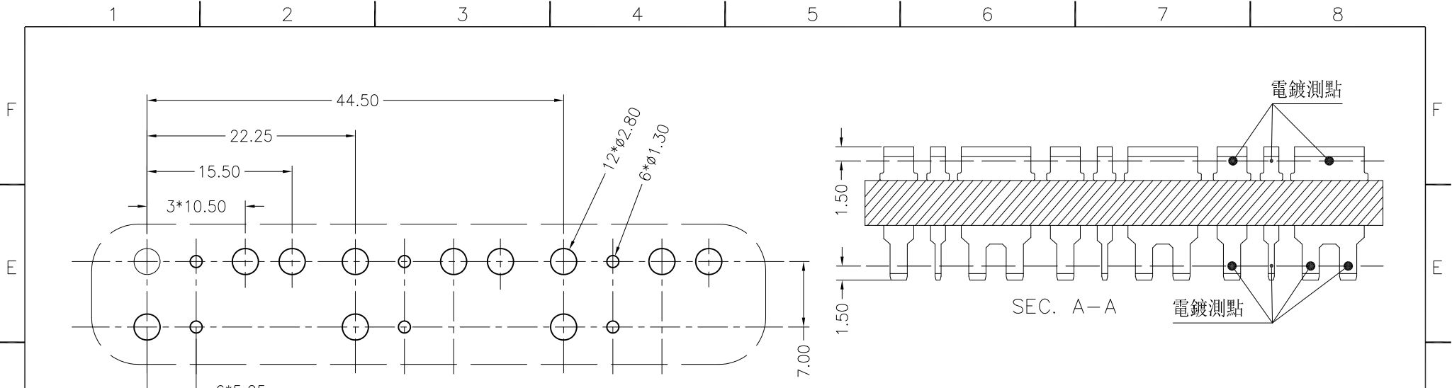
PCB 插板參考尺寸
