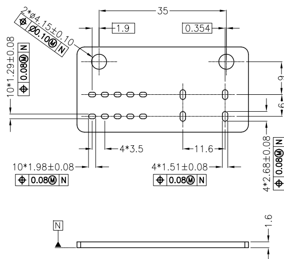
电路板参考尺寸
