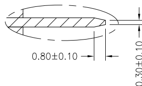
DETAIL F 2:1
